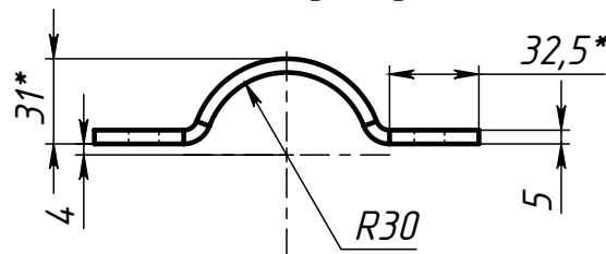
Поз.8 (Полухомут)
