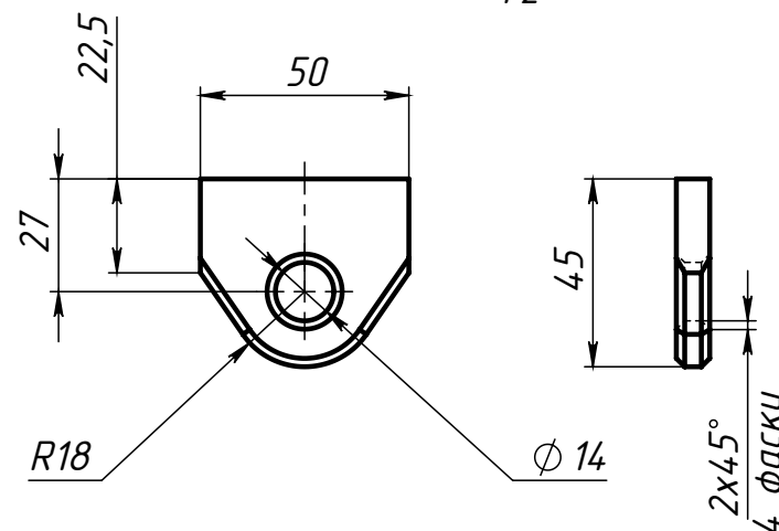
Поз.1 (Проушина) 1:2
