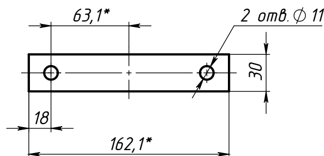
Поз.8 (Полухомут) развертка
