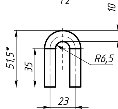
Поз.3 (Ушко) 1:2
